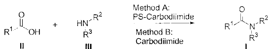
Scheme 1a
