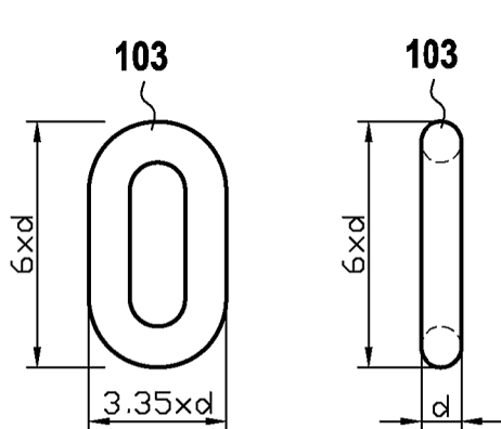
FIG. 2A FIG. 2B (prior art)
