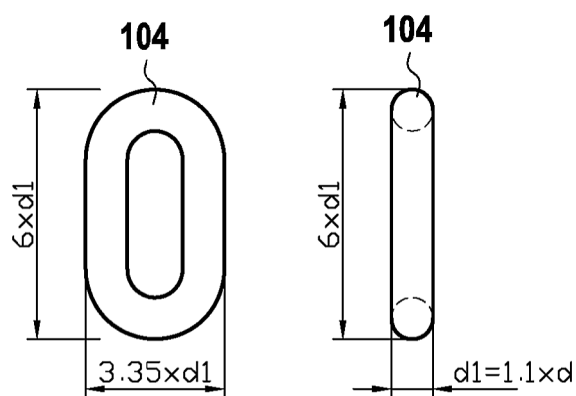
FIG. 3A FIG. 3B (prior art)
