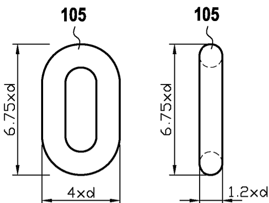
FIG. 4A FIG. 4B (prior art)
