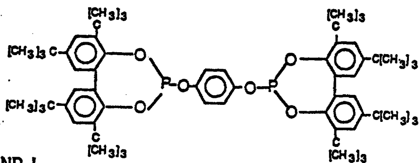
LIGAND J
