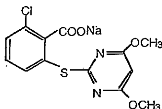
pyriithiobac-sodium
