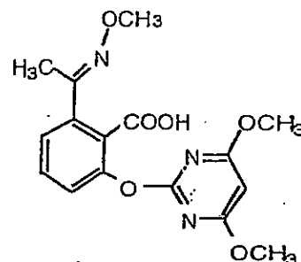
pyriminobac
