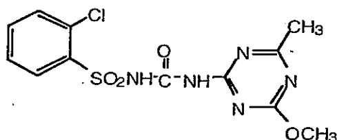
chlorsulfuron
