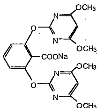
bispyribac-sodium
