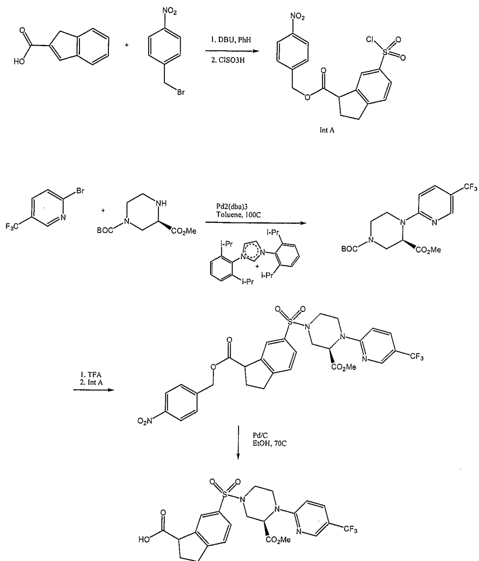
Scheme VI
