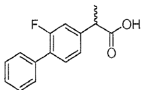
flurbiprofen
