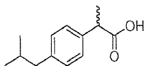
ibuprofen
