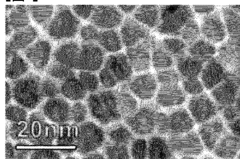
Co-Pt-Cr-TiO 2 -SiO 2
