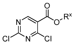
(IIId)
