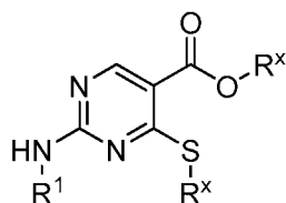
(IId),
