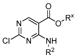
(IIId),
