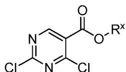
(IIf),
