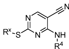
(VIIb),
