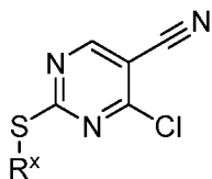
(Ig)
