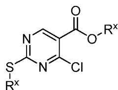
(Ie),
