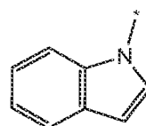
indol-1-yl
