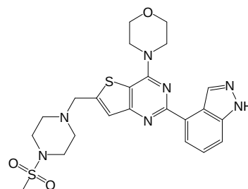
GDC-0941
