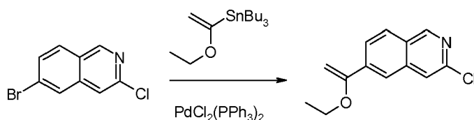
Compound 2e
