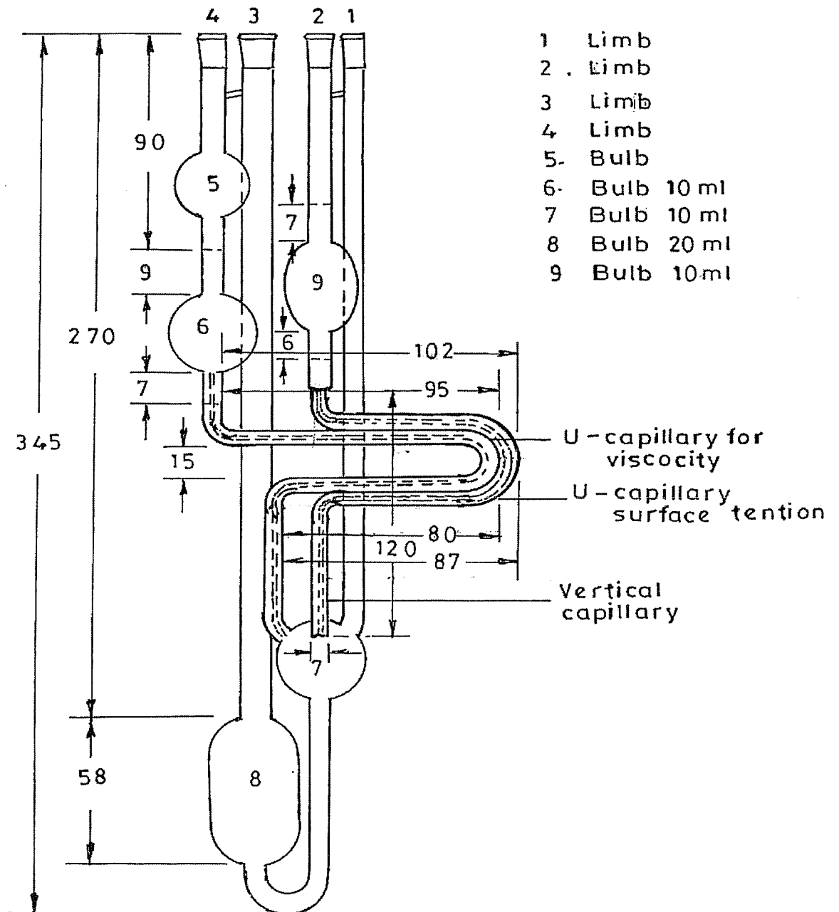
SURVISMETER - TYPE 2
