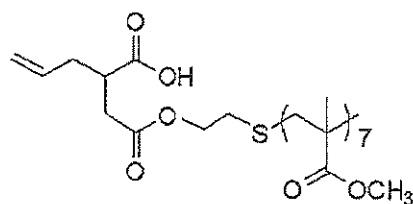
Macromonomer E5
