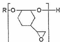
EHPE-3150
