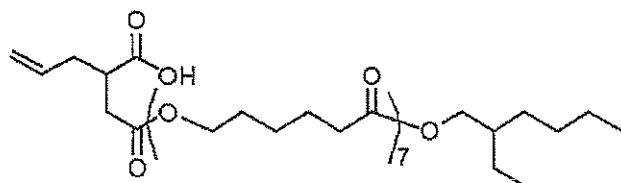
Macromonomer A5
