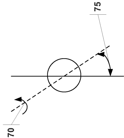
FIG. 9C (Side View)
