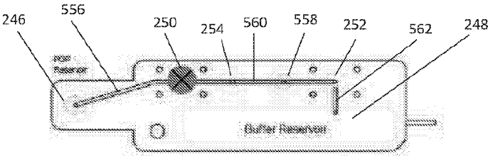
FIG. 14C
