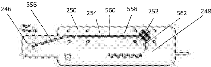
FIG. 14A
