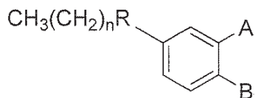
Formula IC
