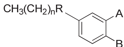
Formula IC
