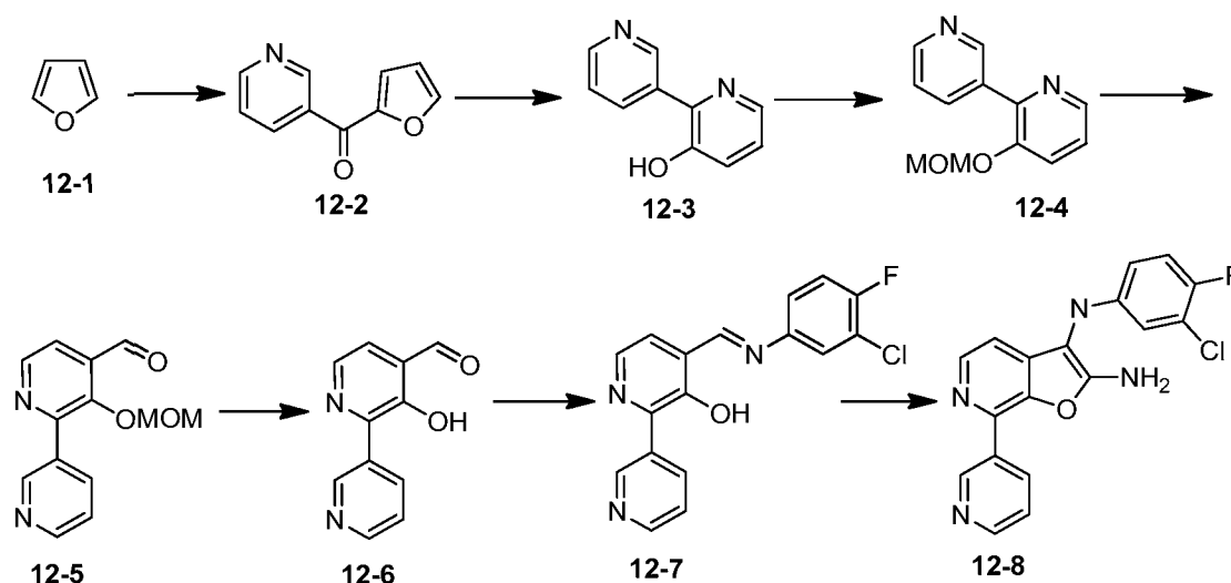
Scheme 12B
