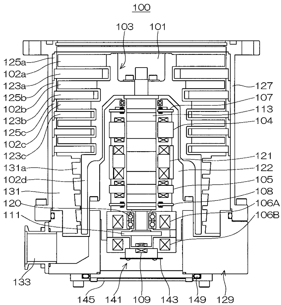
[図1]
