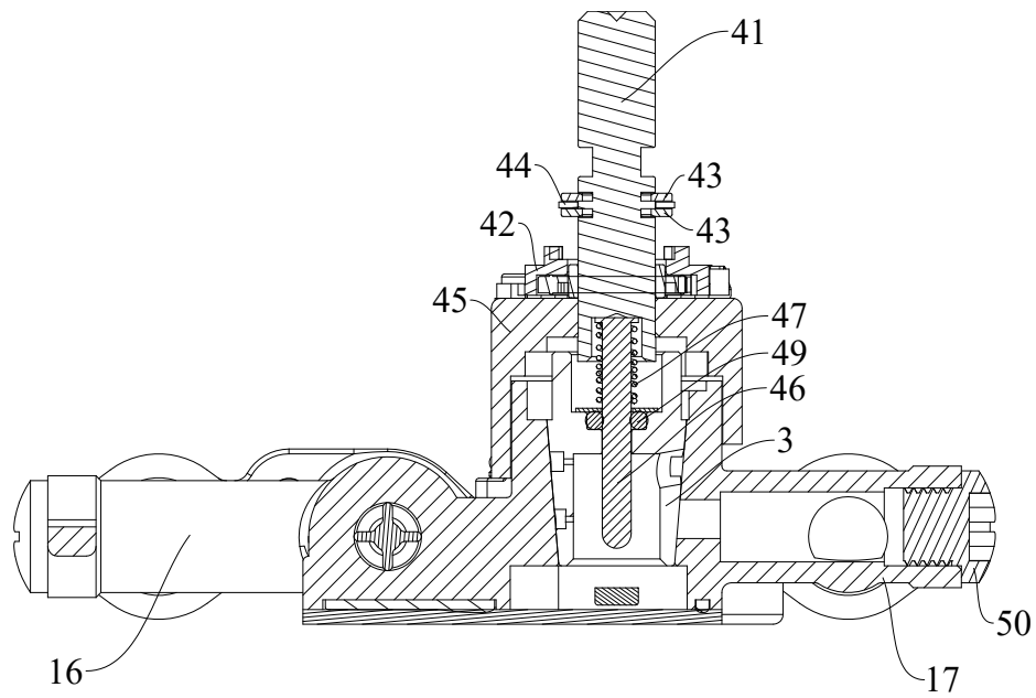
C-C FIG. 5
