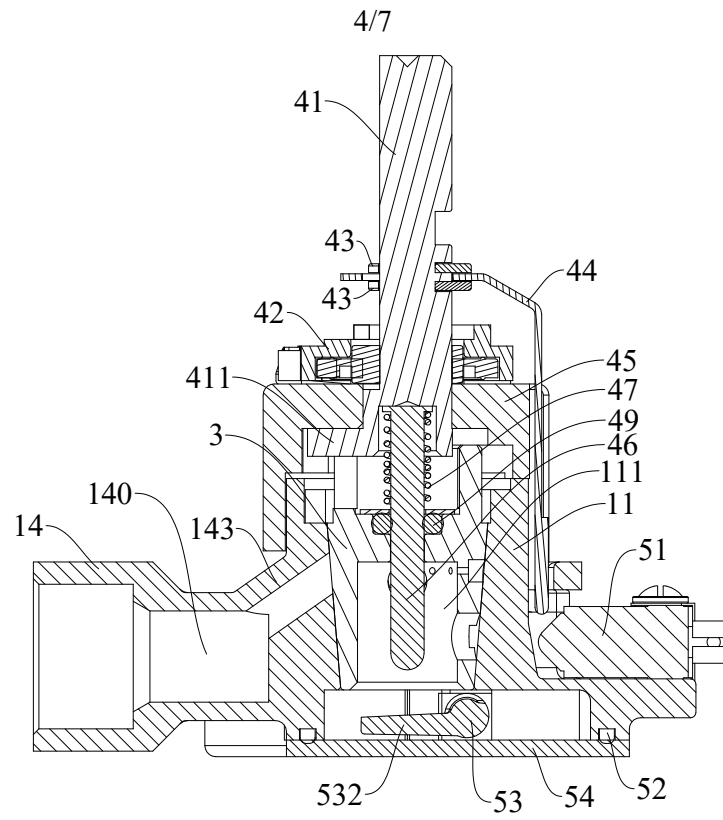
A-A FIG. 4
