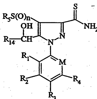
(VIII)
