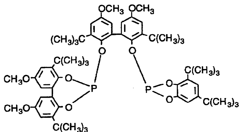
Ligand N
