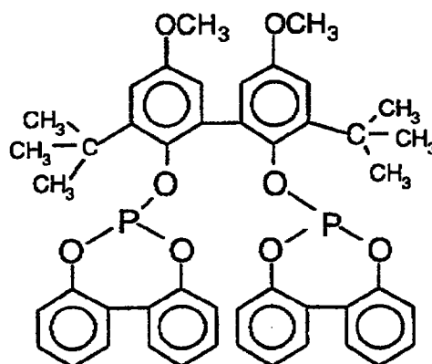
Ligand D
