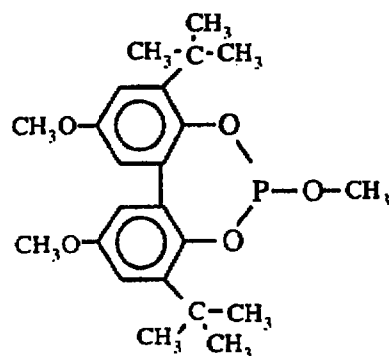
Ligand B
