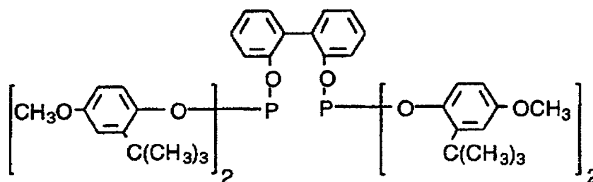
Ligand V
