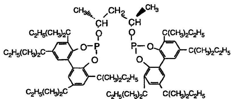
Ligand G
