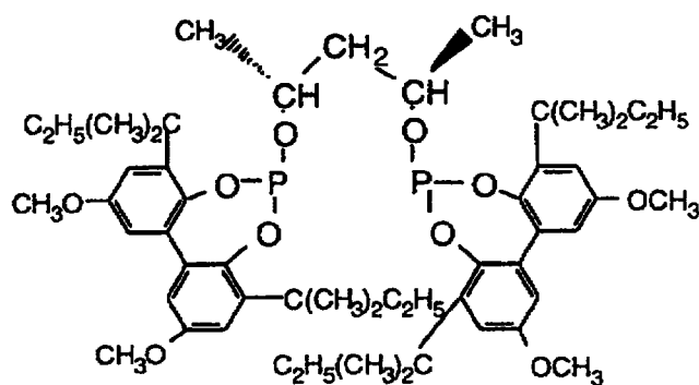
Ligand I
