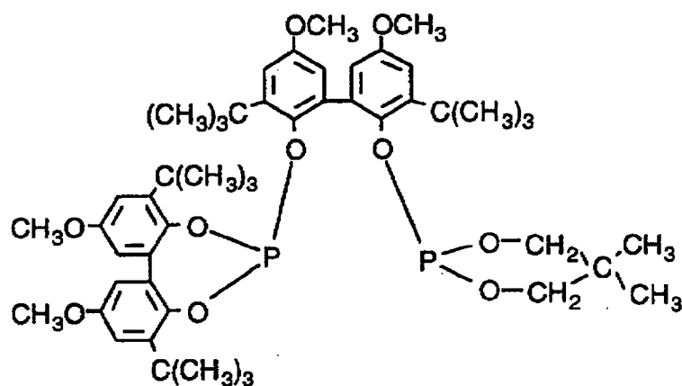
Ligand P
