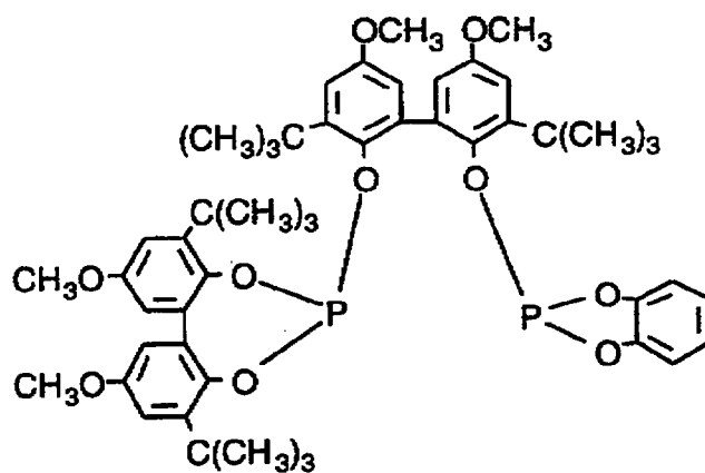
Ligand O
