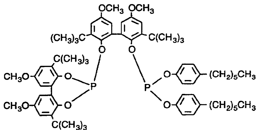
Ligand Q
