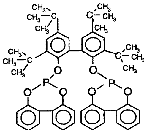
Ligand F
