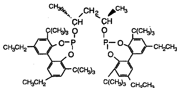
Ligand L
