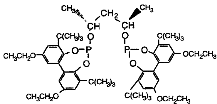
Ligand K
