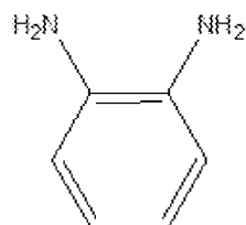
1,2-benzenediamine,
