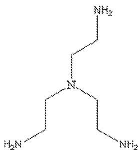
N,N-bis(2-aminoethyl)-1,2-ethanediamine,
