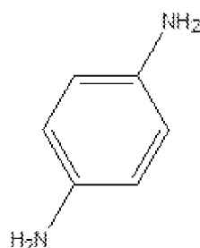
1,4-benzenediamine .
