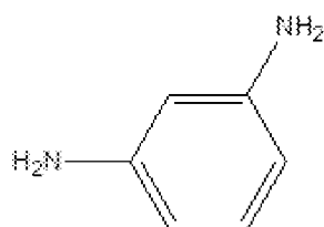
1,3-benzenediamine , and
