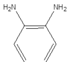
1,2-benzenediamine,
