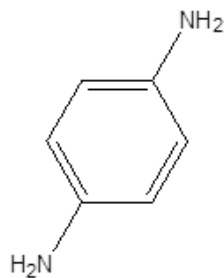
1,4-benzenediamine .
