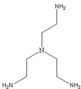
N,N-bis(2-aminoethyl)-1,2-ethanediamine,
