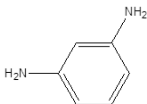
1,3-benzenediamine , and
