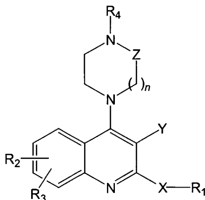
(Ib)
