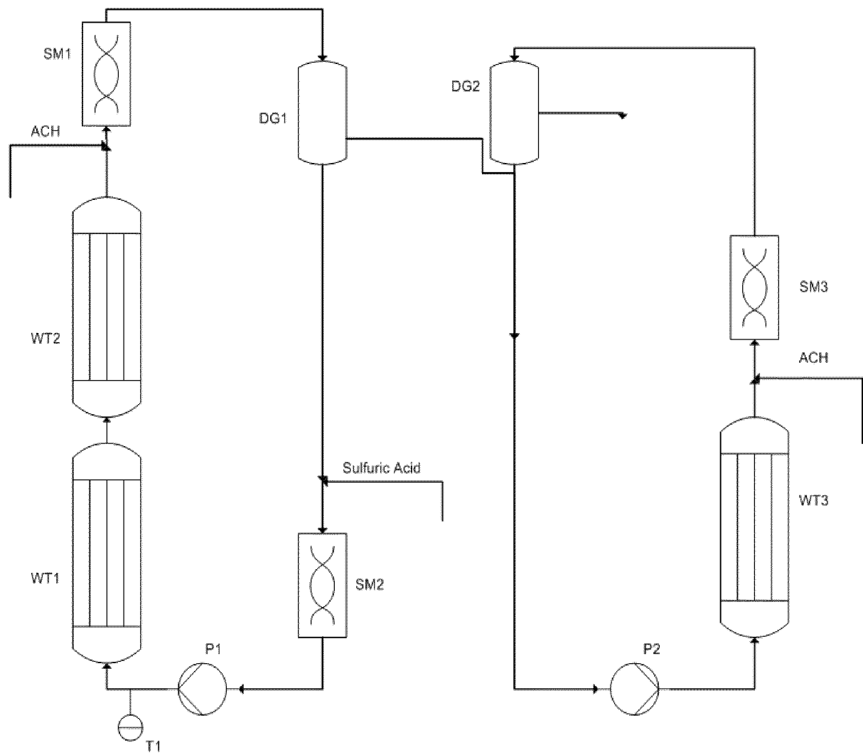
Fig. 2 Fließdiagramm Vergleichsbeispiele 1-4
