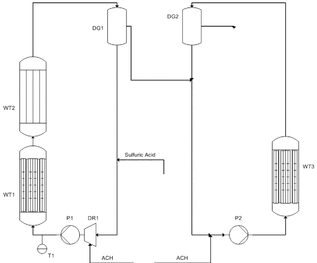
Fig. 3: Fließdiagramm Beispiele 1-4
