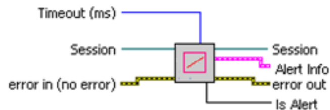
GetAlert(RTSub).vi
