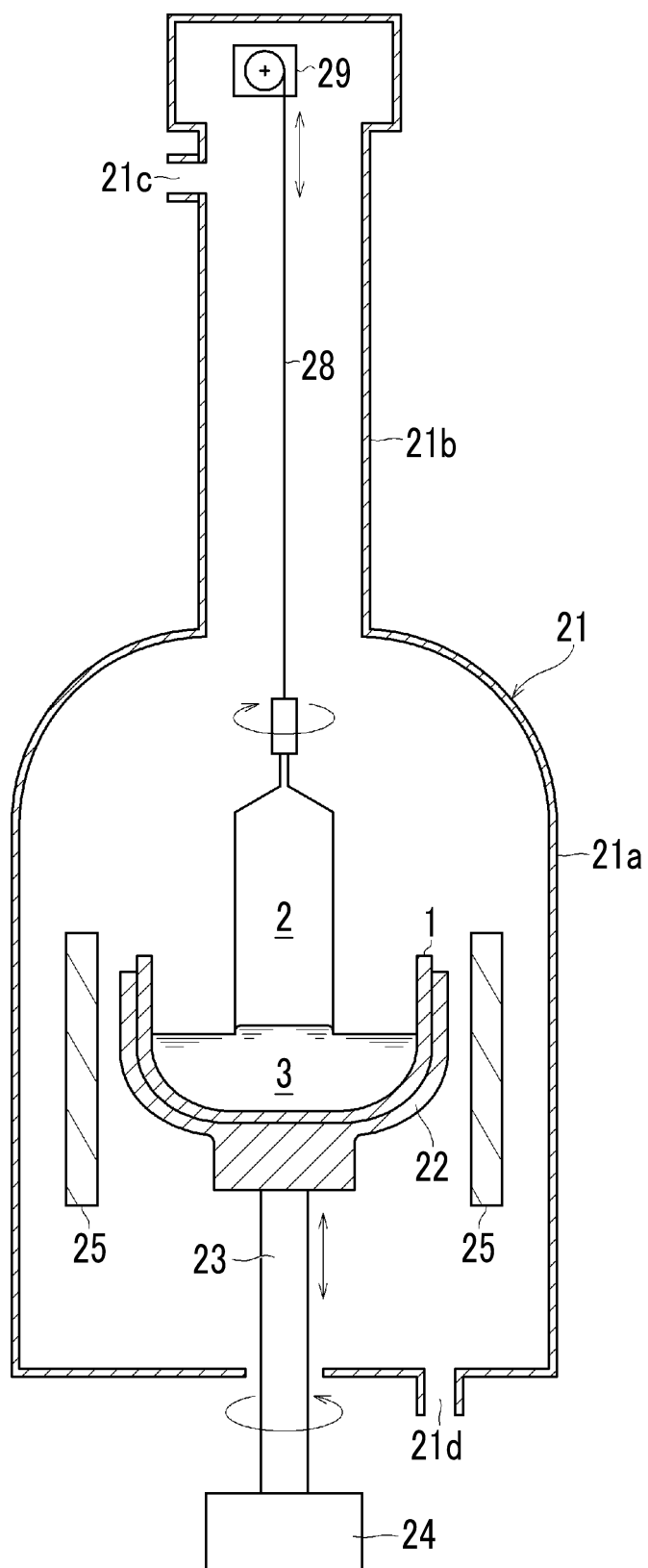
7/7 FIG. 7 20
