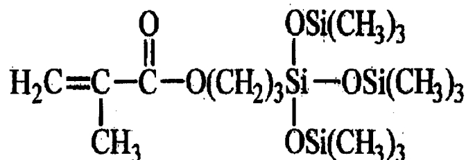
Tris
