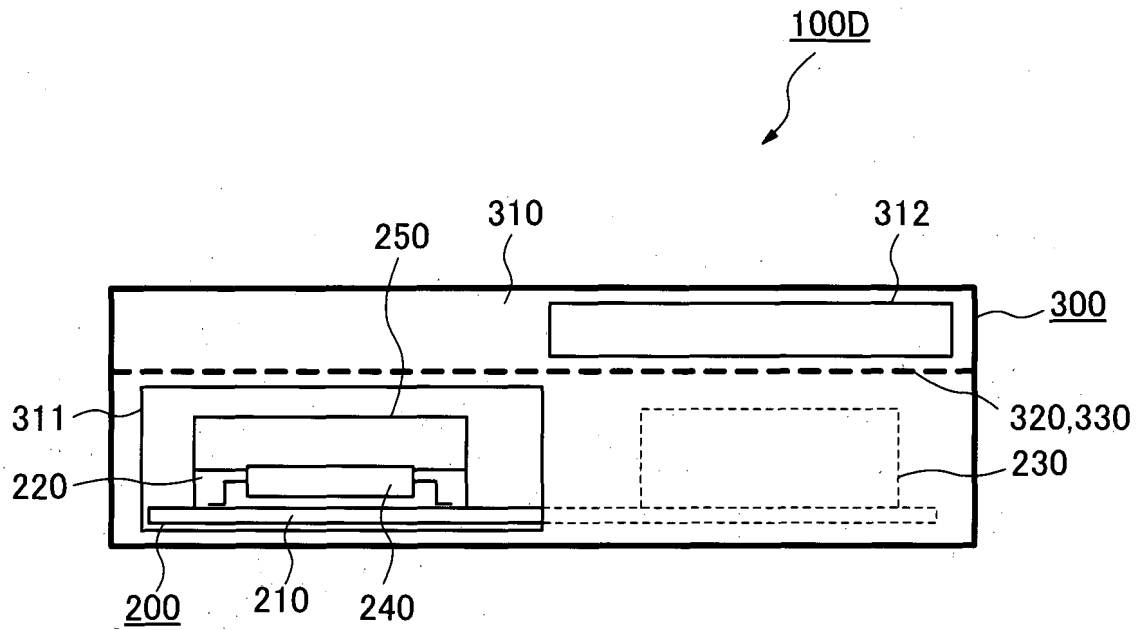
矢視J
