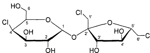
SUCRALOSE
