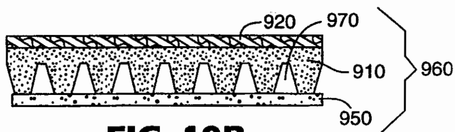
FIG. 10B
