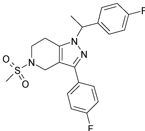
enantiomer 1
