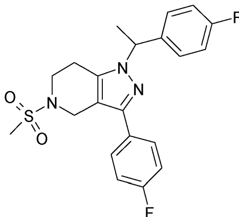
enantiomer 2
