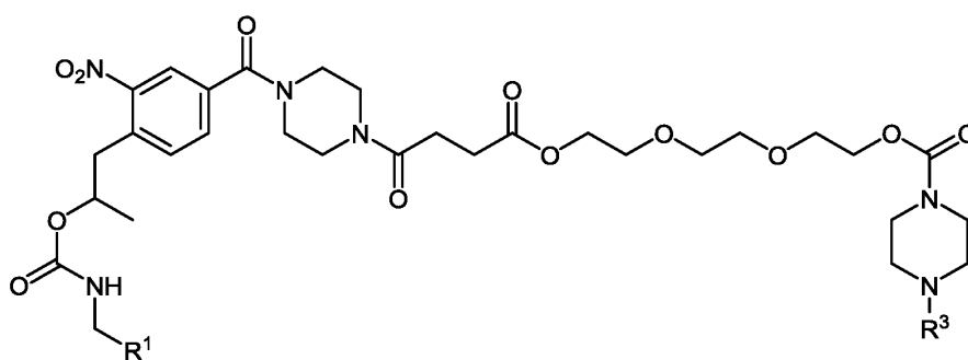
(A3);
