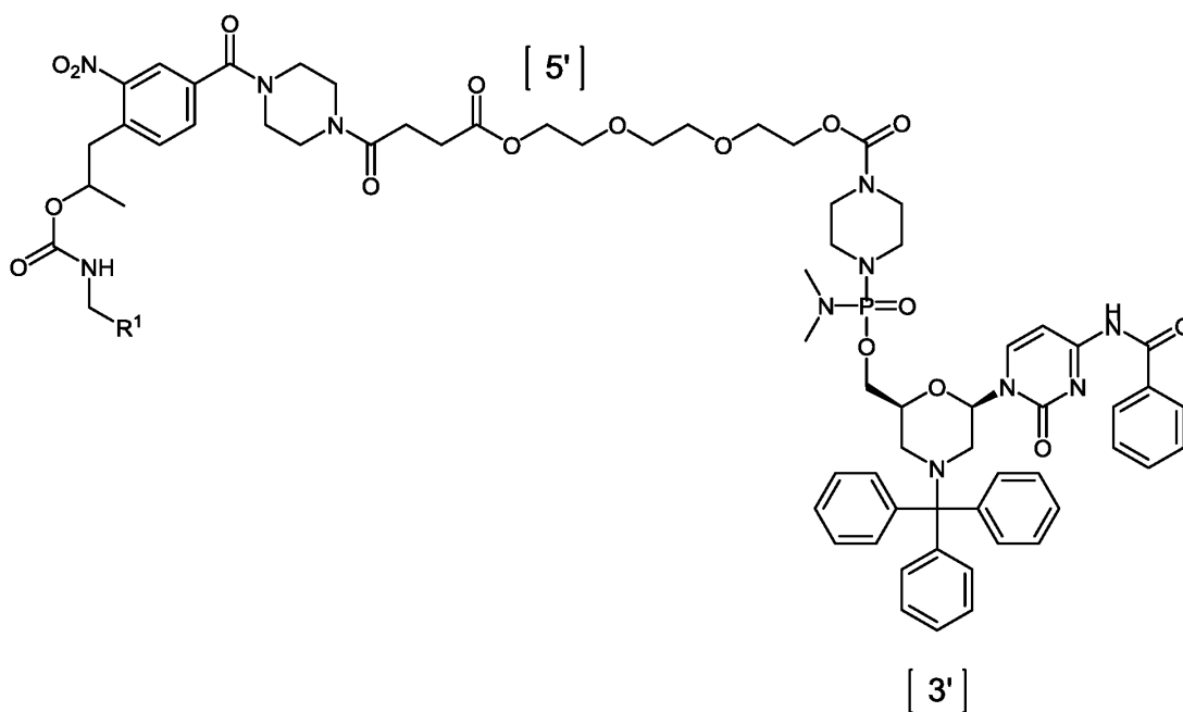
(Va),
