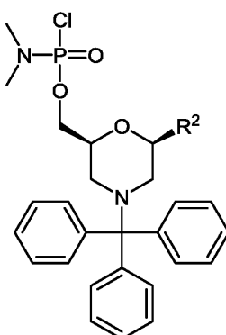
(VIIIa);
