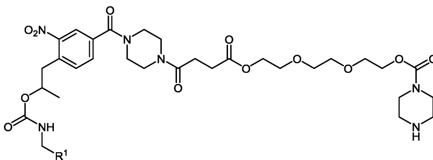
(IV);
