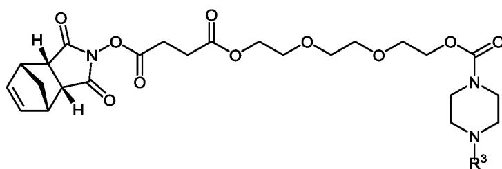
(A2);
