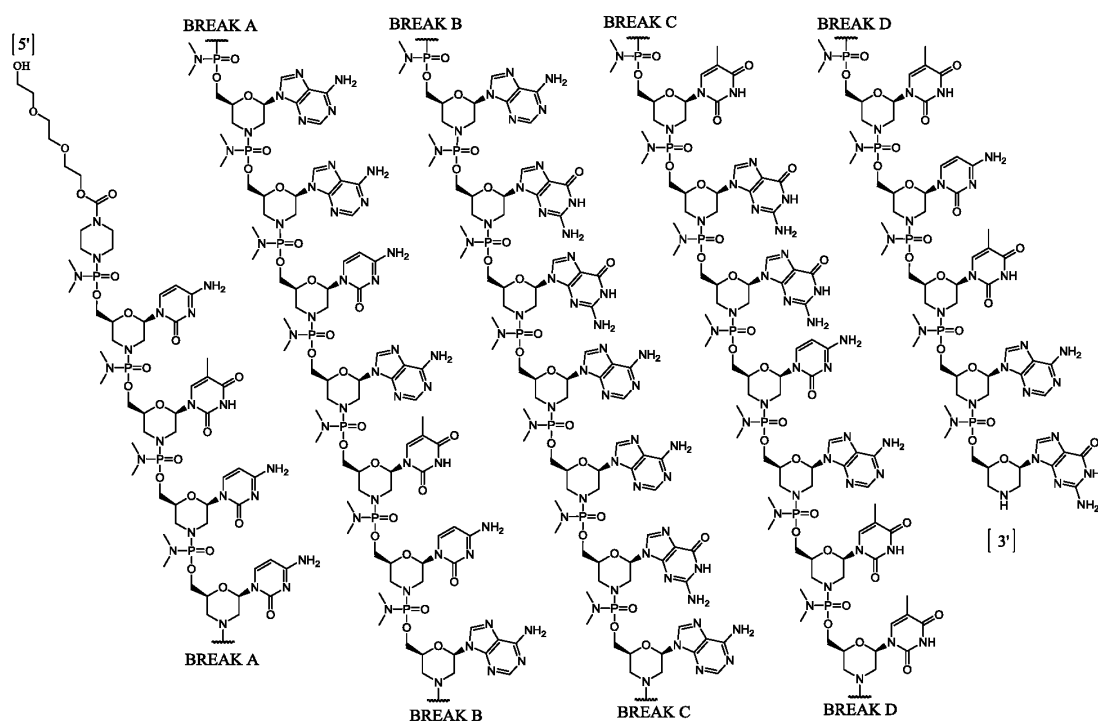
(XII).
