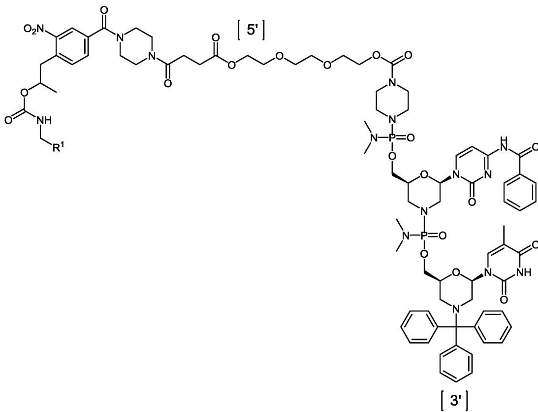
(VIIa),
