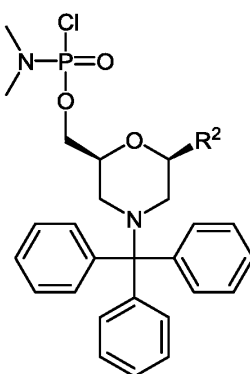
(VIIIa);
