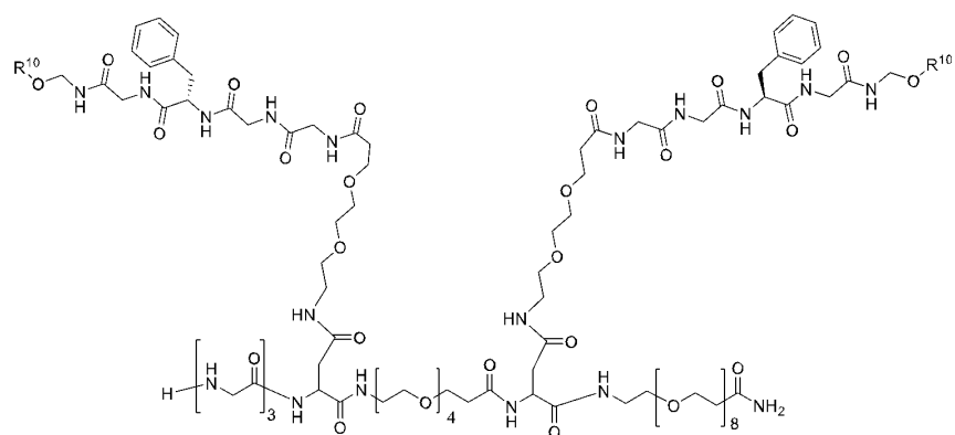
(I-b-0-1)
