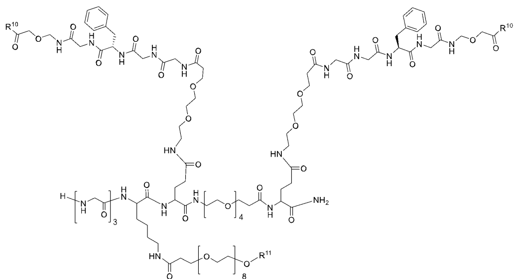
(I-b-1-9).
