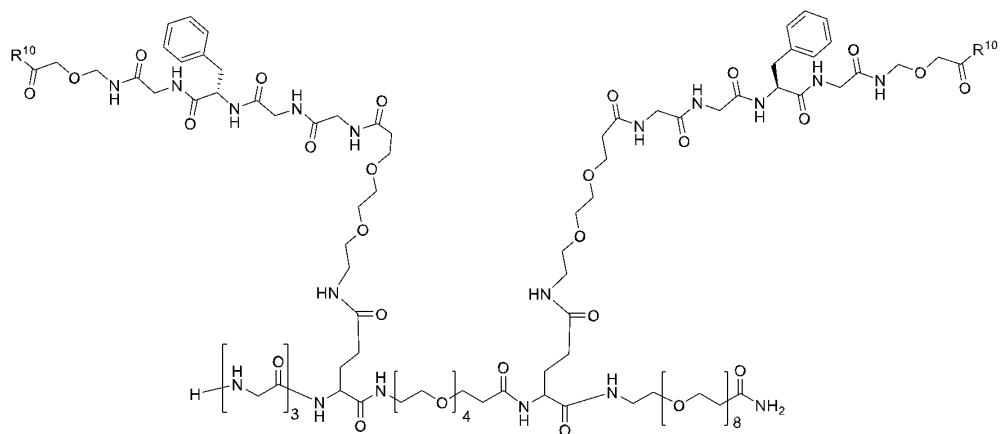
(I-b-0-9).
