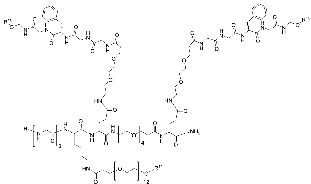
(I-b-1-10)
