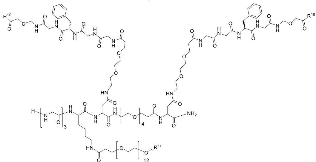
(I-b-1-6).
