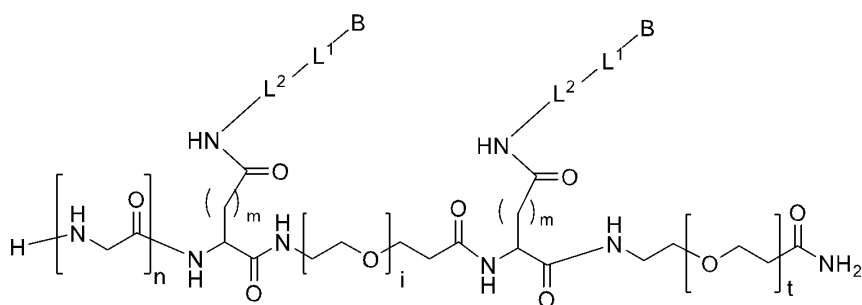
(I-b-0).
