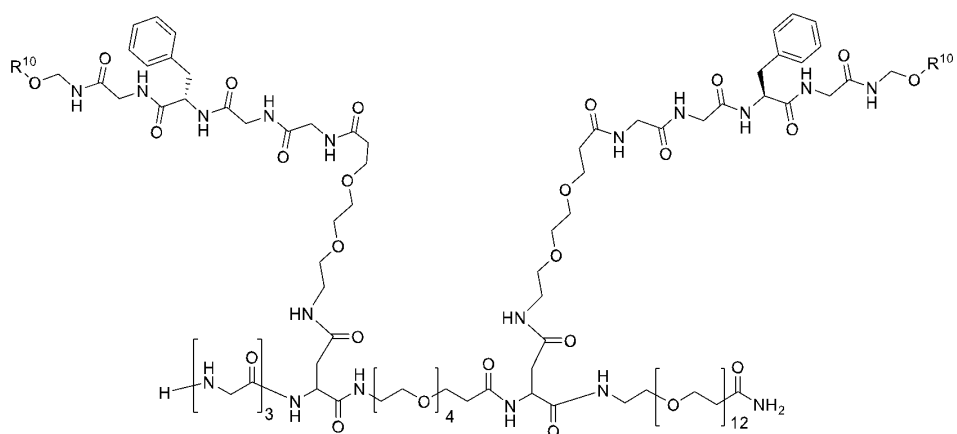
(I-b-0-4)
