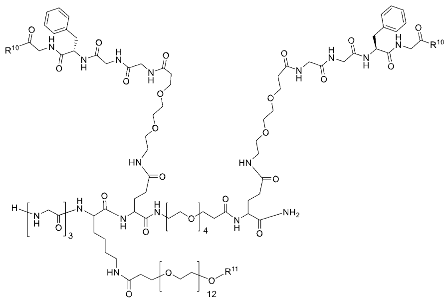
(I-b-1-11)
