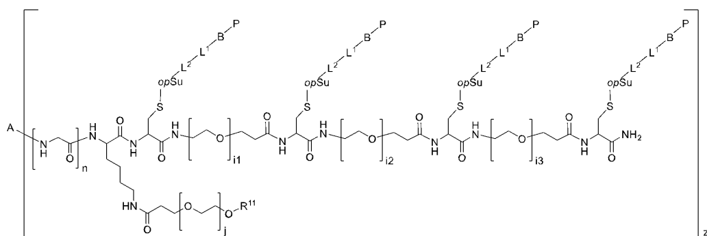
(conjugate III-a-1-4).
