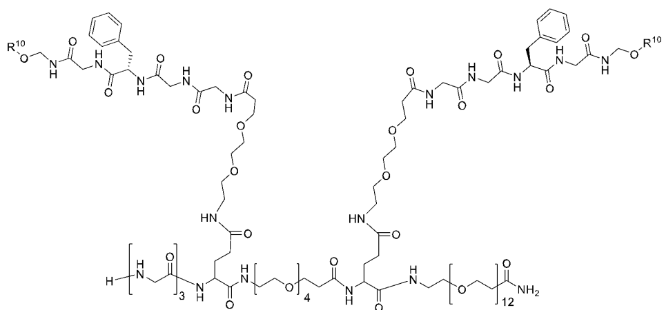
(I-b-0-10)
