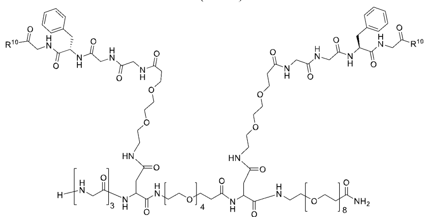
(I-b-0-2)
