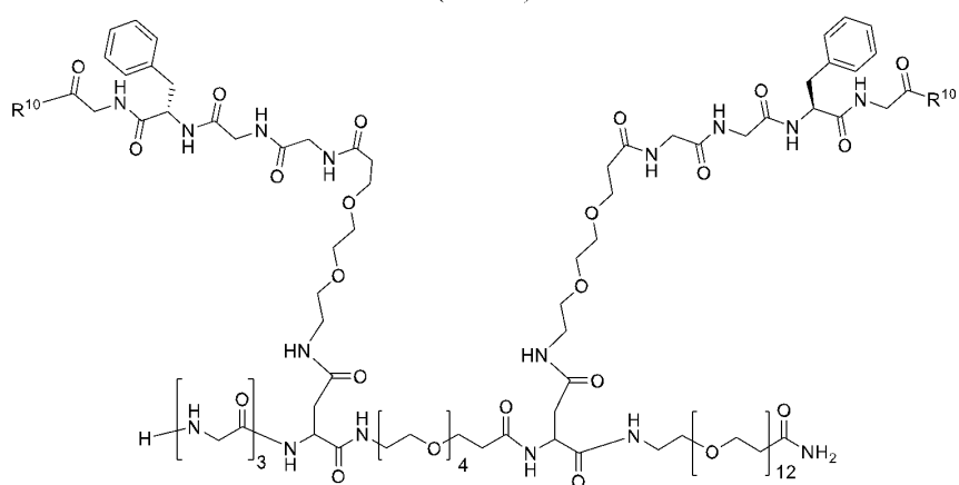
(I-b-0-5)
