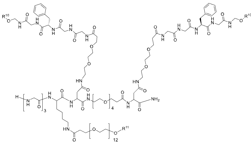
(I-b-1-4)
