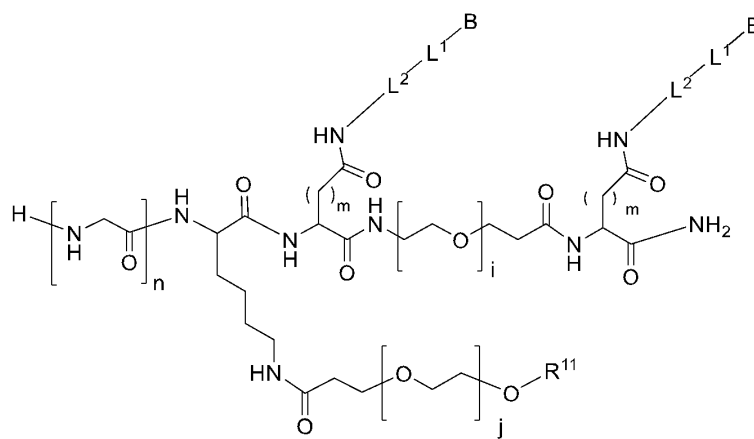
(I-b-1).
