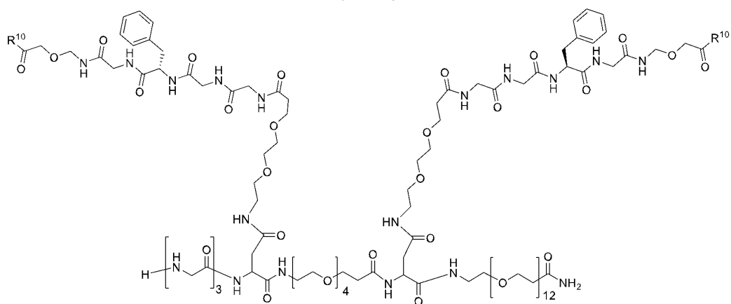
(I-b-0-6).
