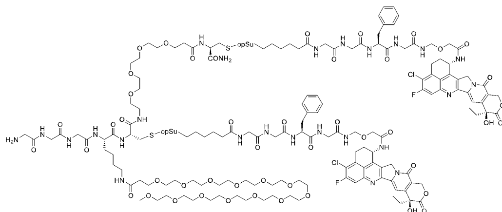
linker-payload 4
