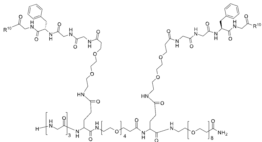
(I-b-0-8)
