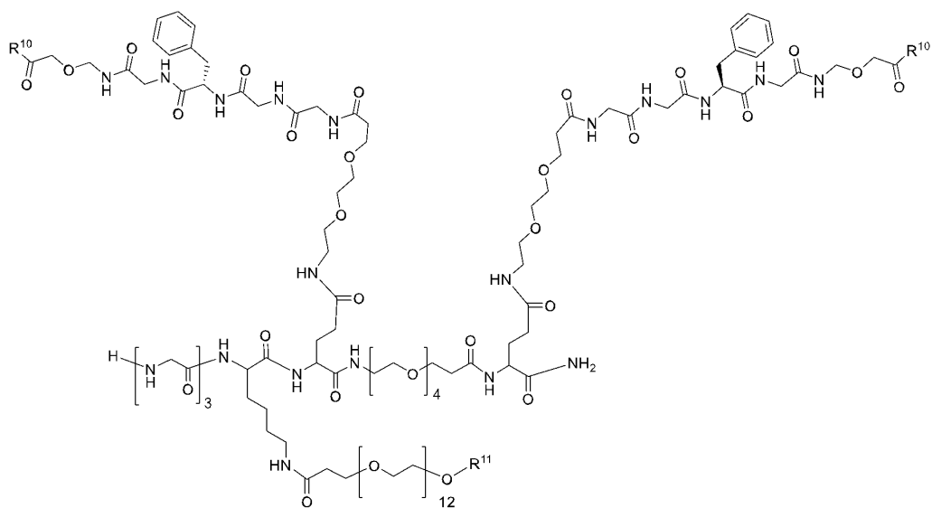
(I-b-1-12).
