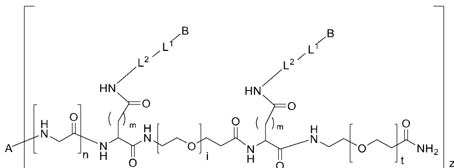
(conjugate III-b-0-1)
