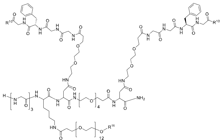
(I-b-1-5)
