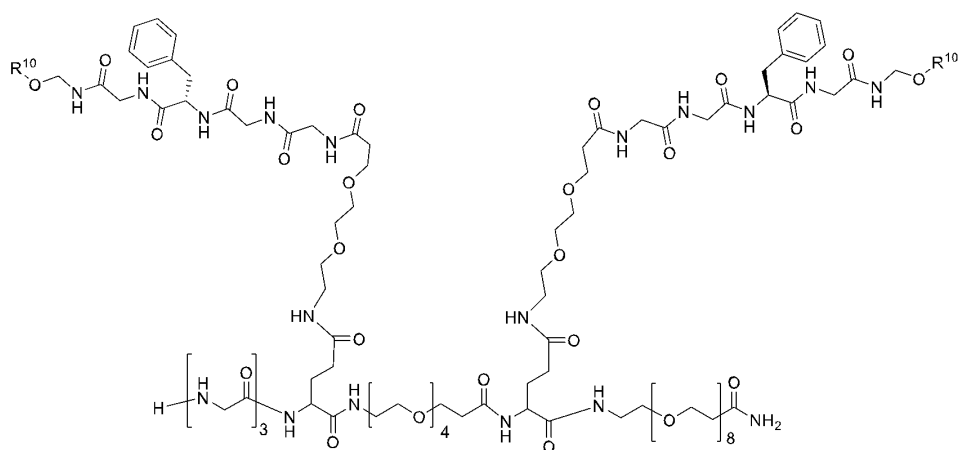
(I-b-0-7)
