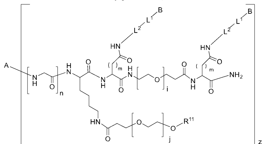
(conjugate III-b-1-1)
