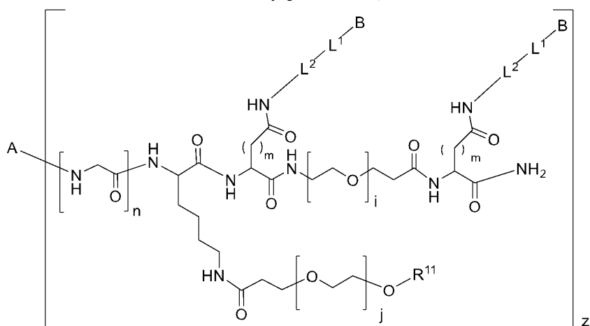
(conjugate III-b-1-1)
