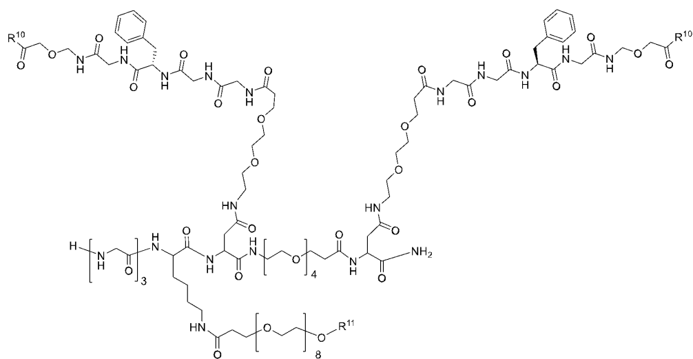
(I-b-1-3).
