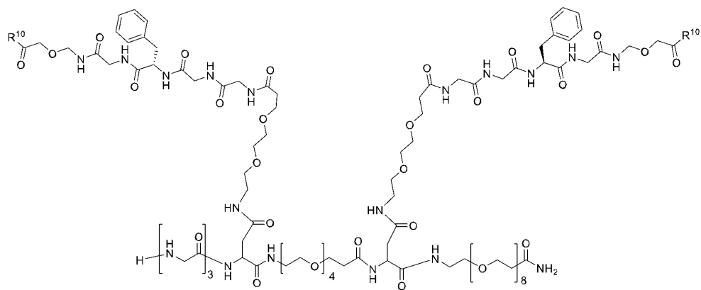
(I-b-0-3).
