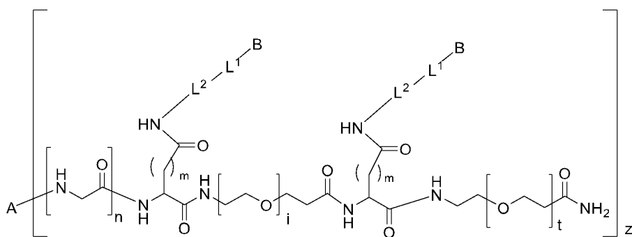
(conjugate III-b-0-1)
