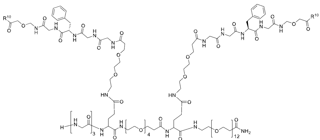
(I-b-0-12).
