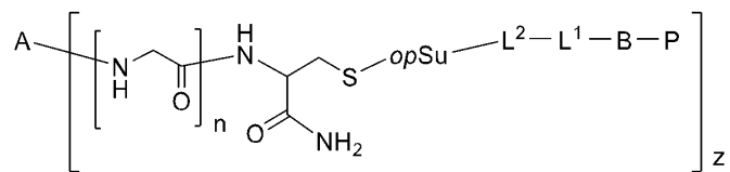
(conjugate III-a-0-1)
