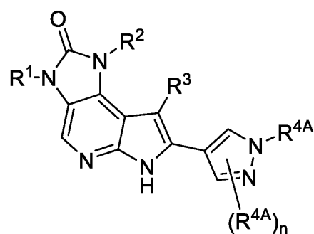
IV
