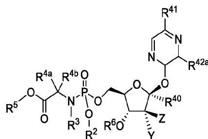
Formula VIId
