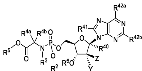
Formula VIIb
