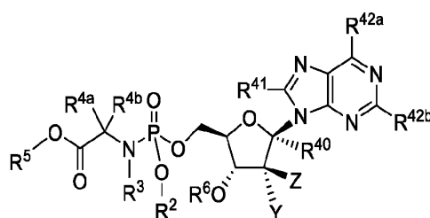
Formula VIIb
