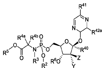
Formula VIId
