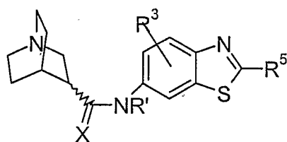
(IIh)
