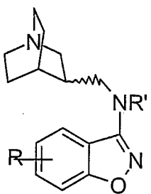
(IVp)
