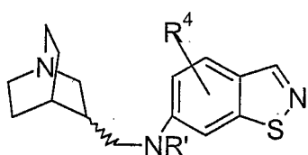
(IVn)
