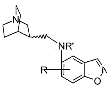
(IVr)
