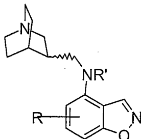
(IVq)
