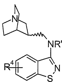
(IVj)
