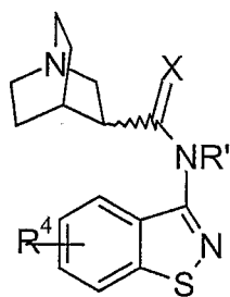
(IIj)
