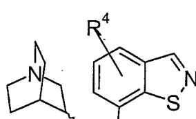
(IVo)
