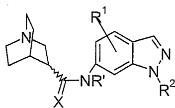
(IIId)
