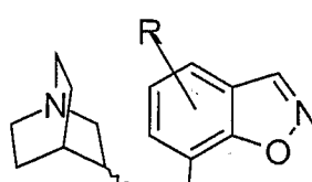
(IVt)
