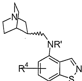
(IVk)
