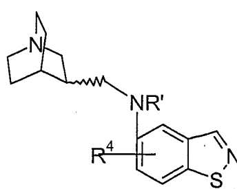
(IVm)
