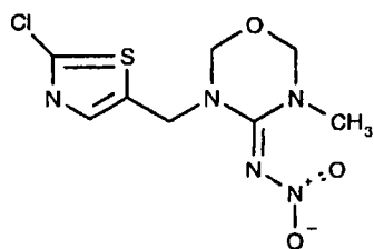
(I, thiamethoxam)
