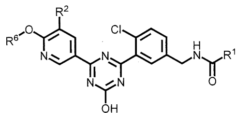
[I-c]
