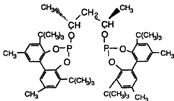
Ligand J
