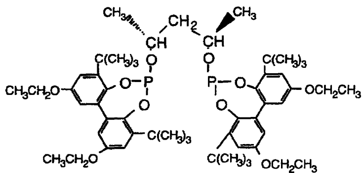
Ligand K
