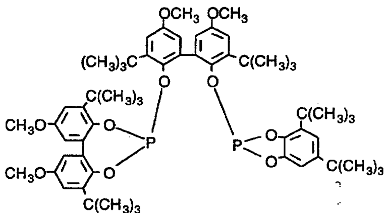
Ligand N
