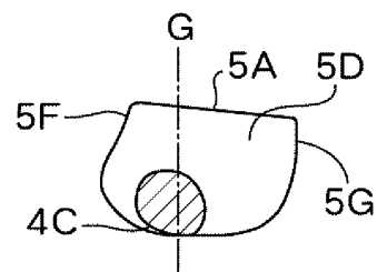
III-III線断面図
