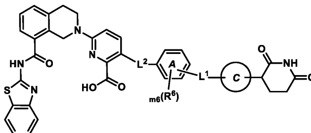
Formula (I-b)
