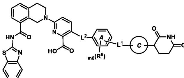
Formula (I-b)
