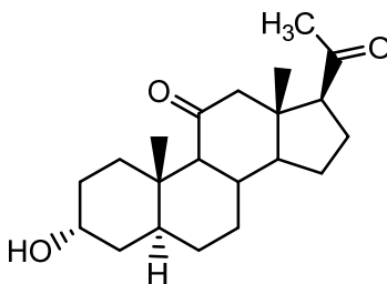
Formula (Ia).
