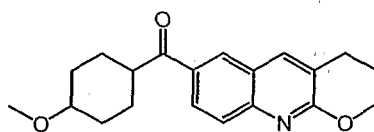
cis
