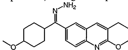
[1α(Z),4α]
