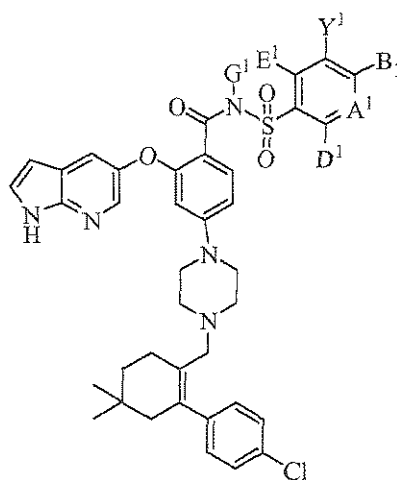
(IIa)
