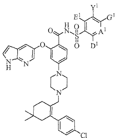
(Ia)
