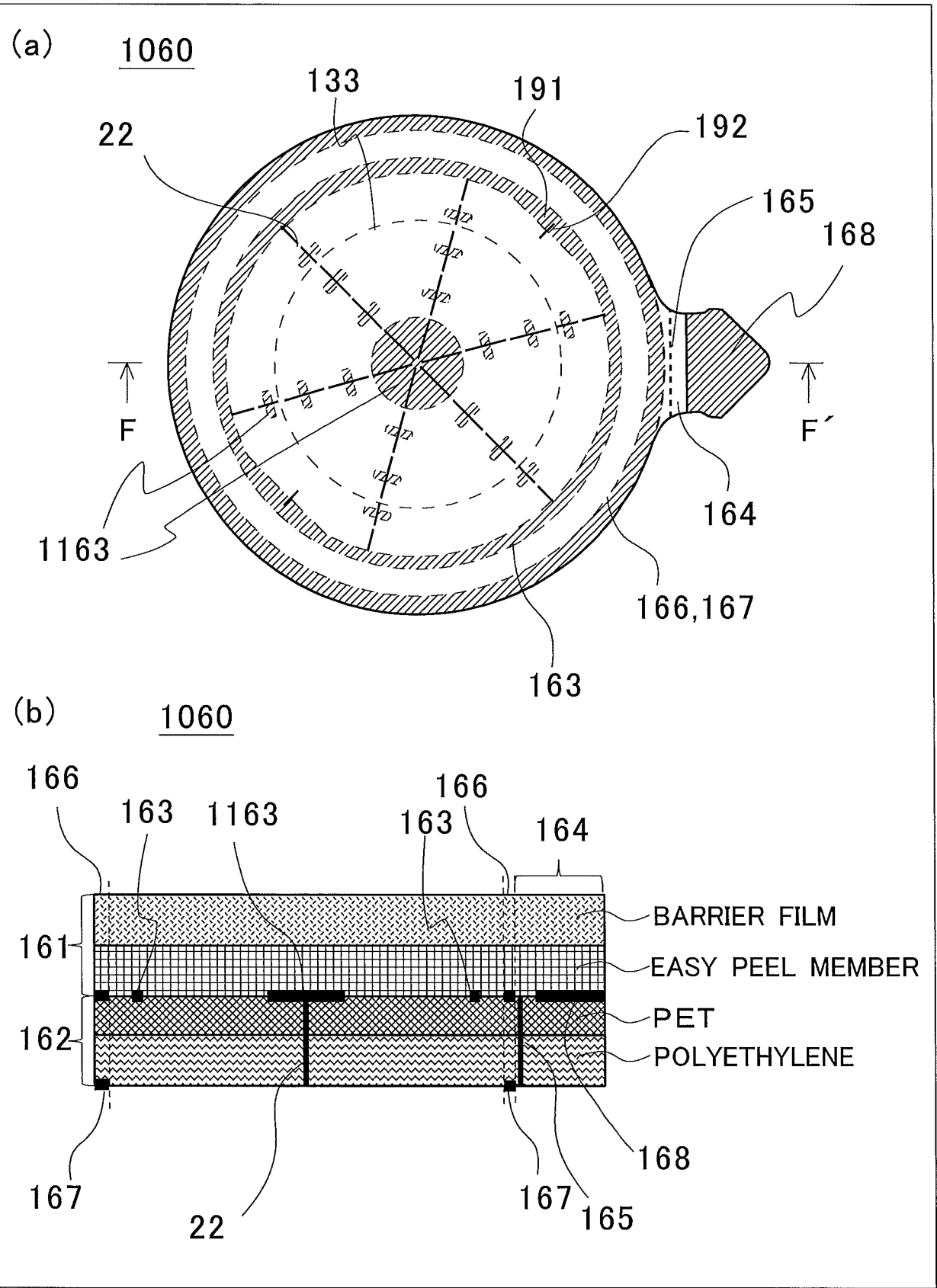
FIG.34
