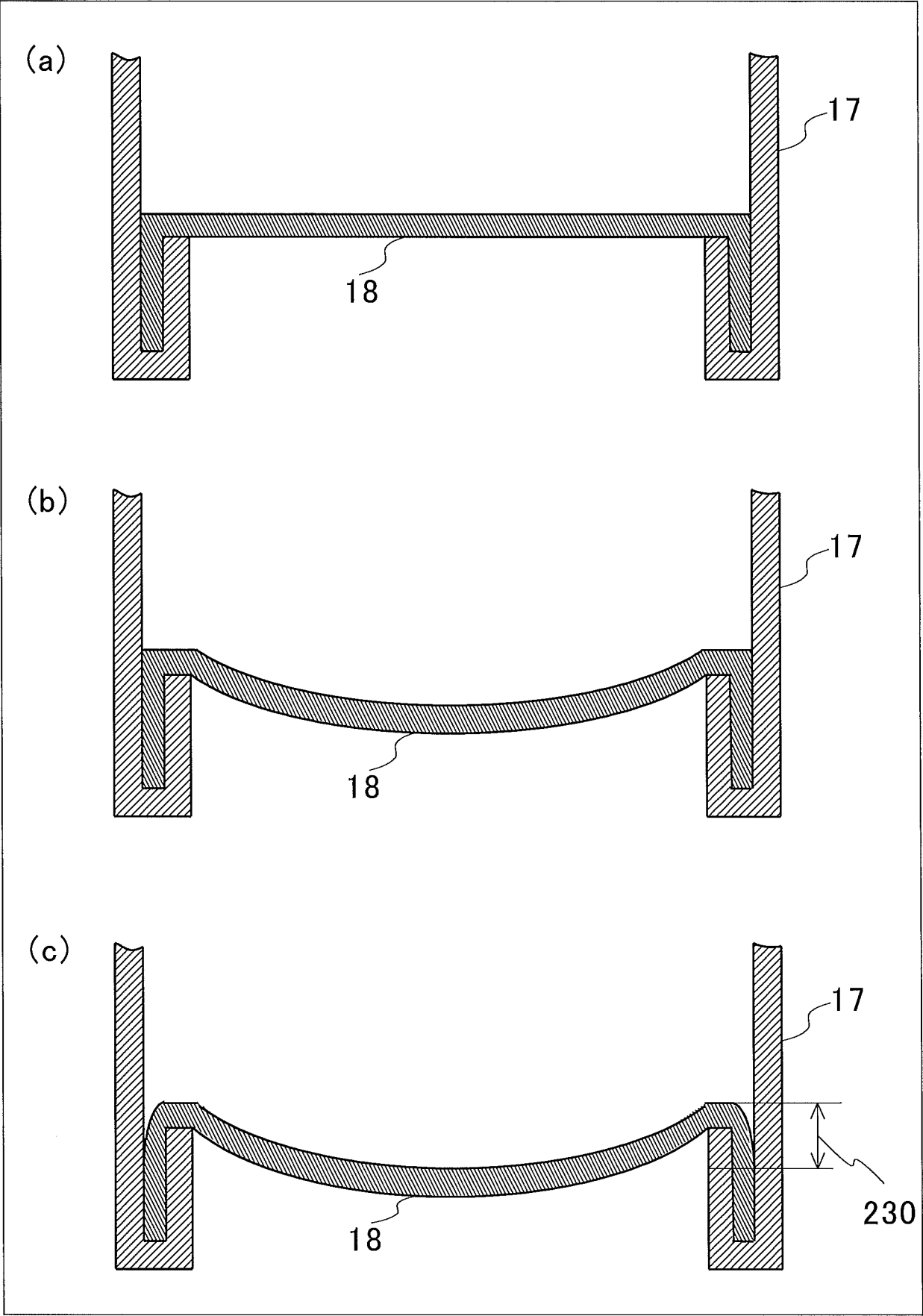
FIG.40
