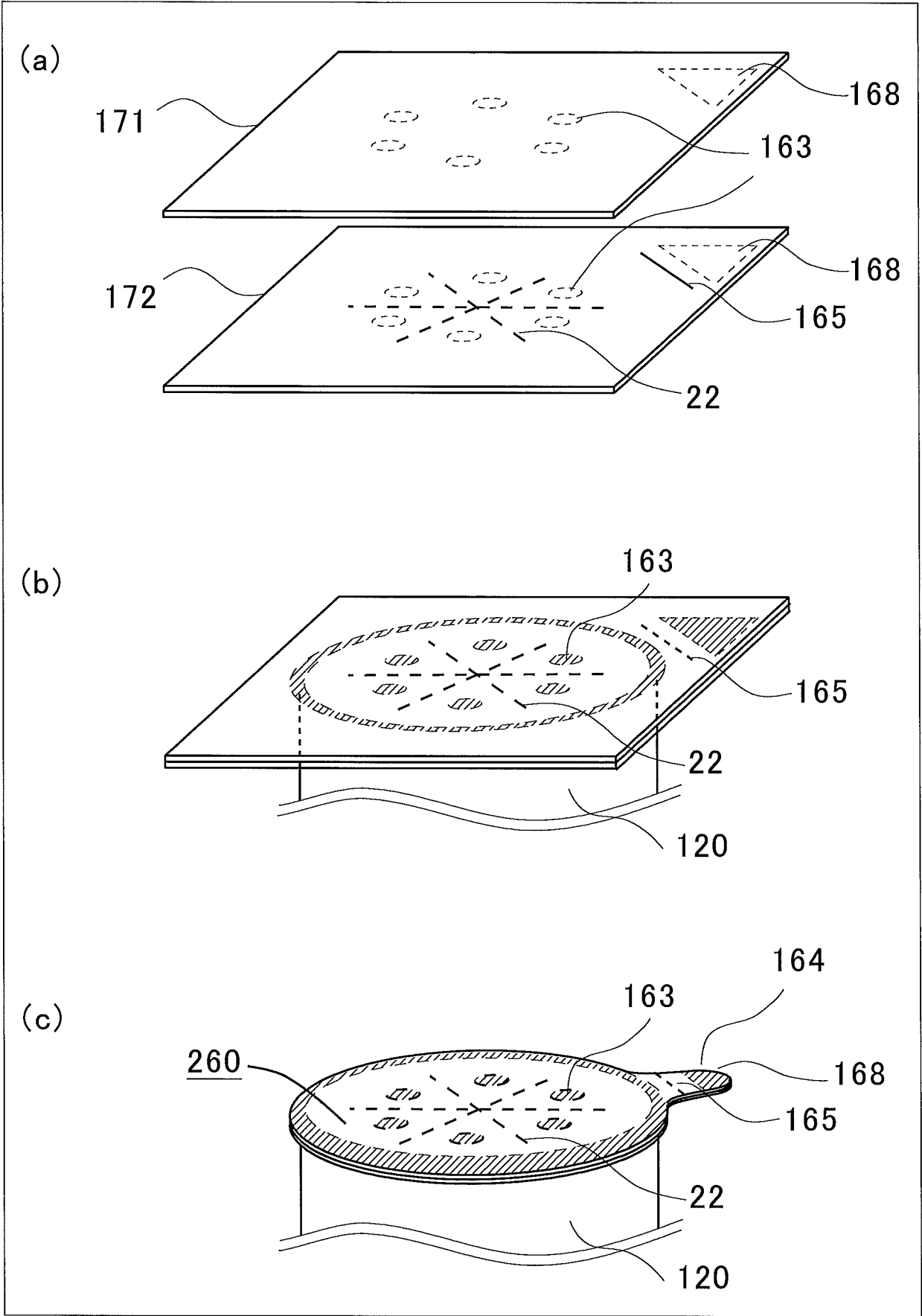
FIG.20
