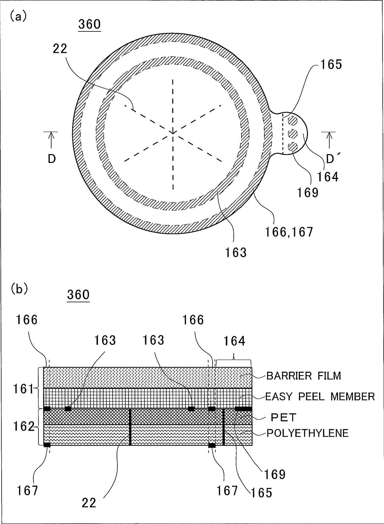
FIG.24
