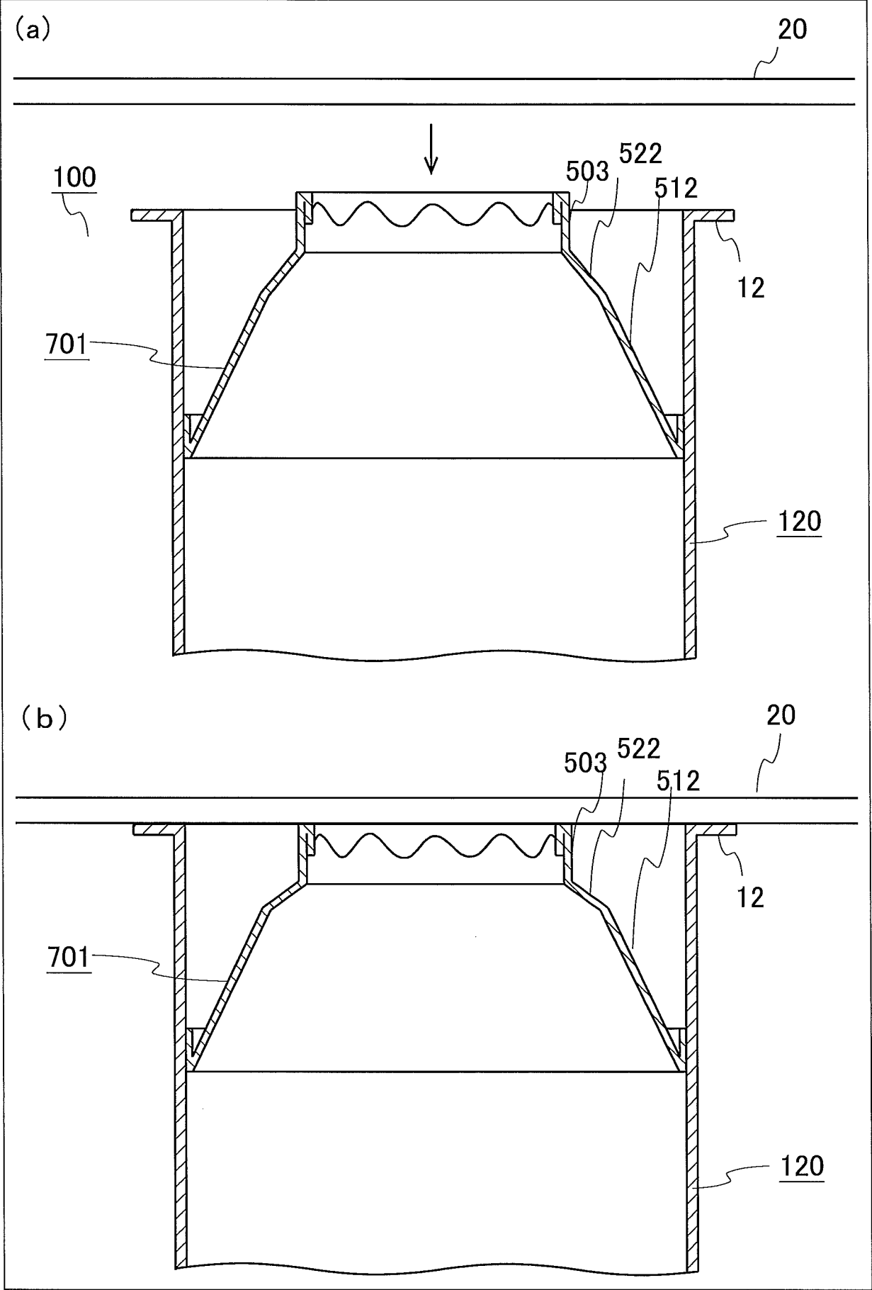
FIG.14
