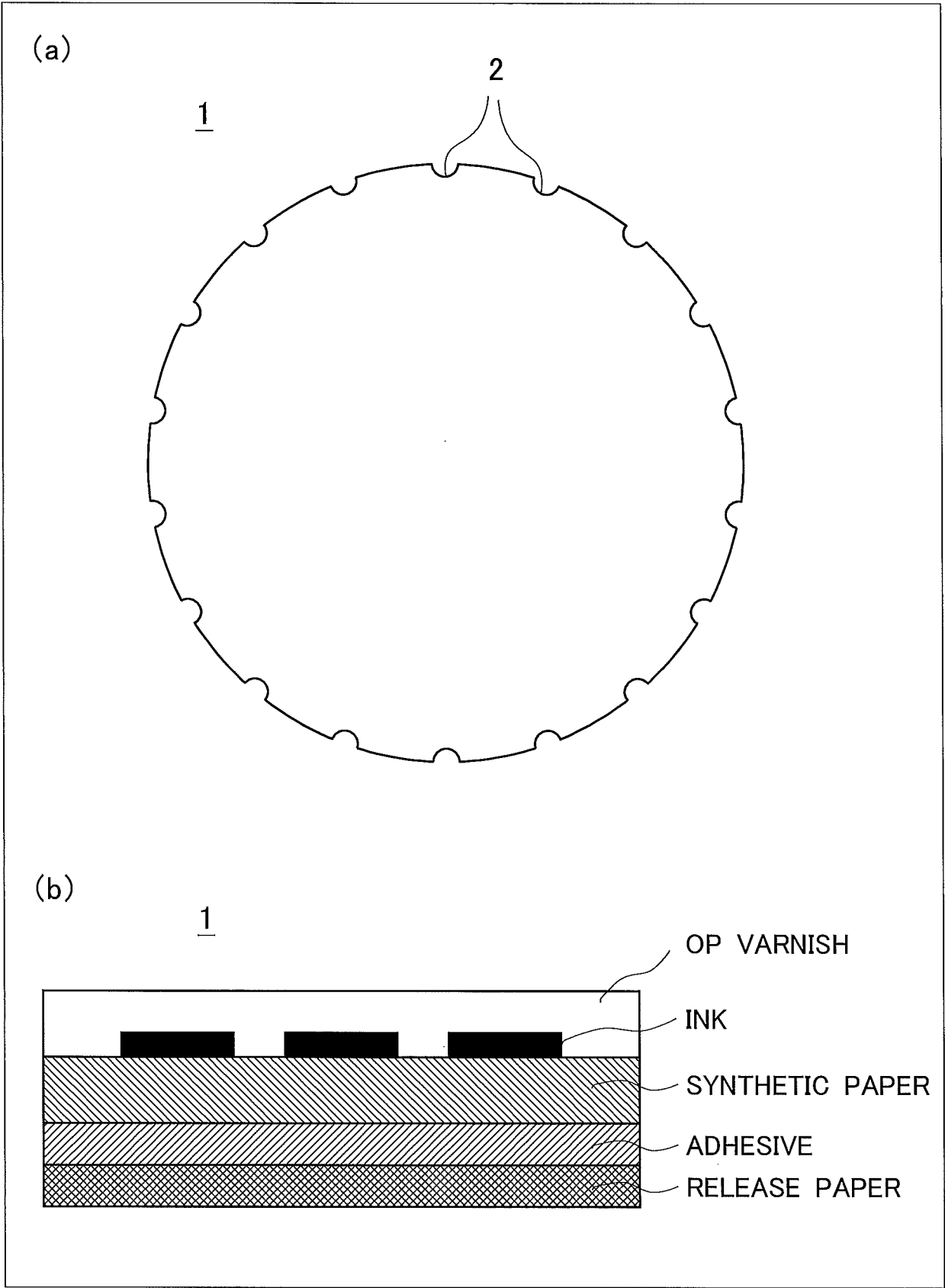
FIG.44
