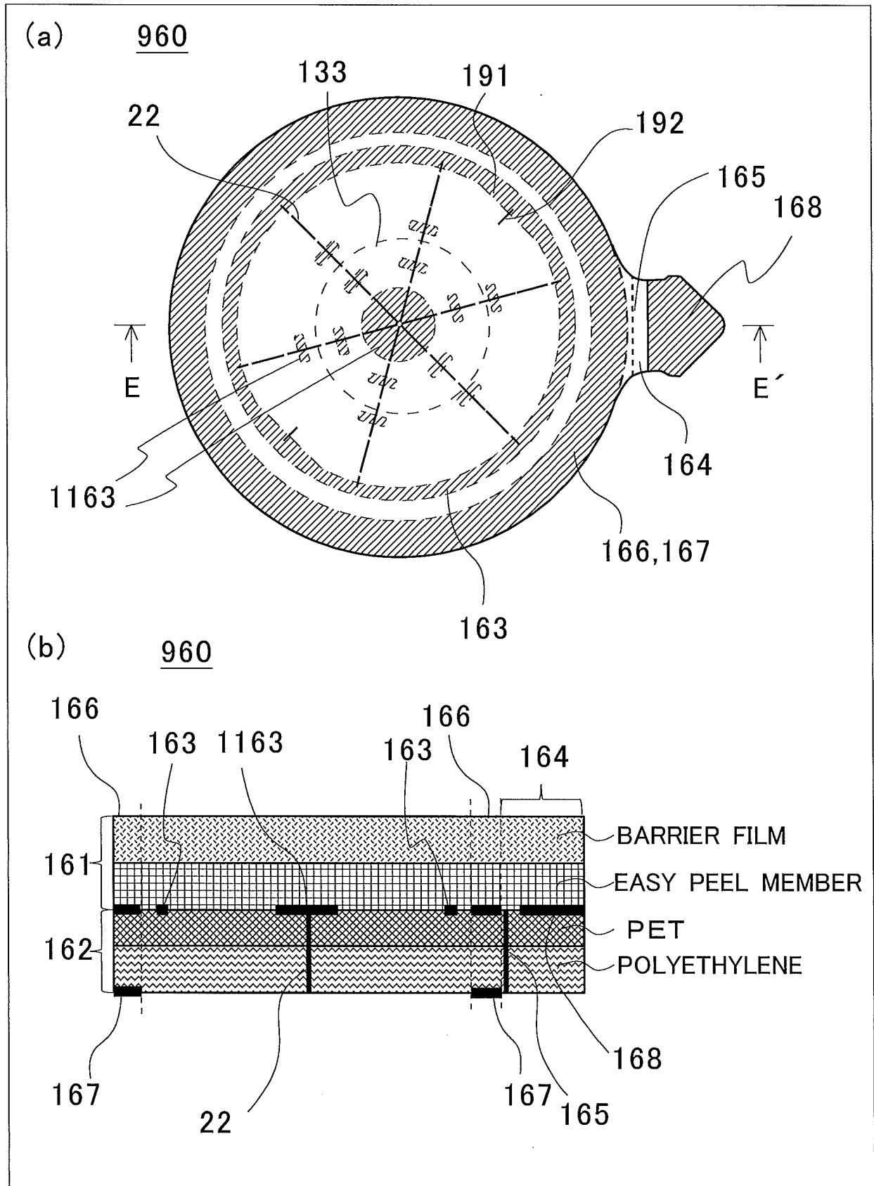
FIG.33
