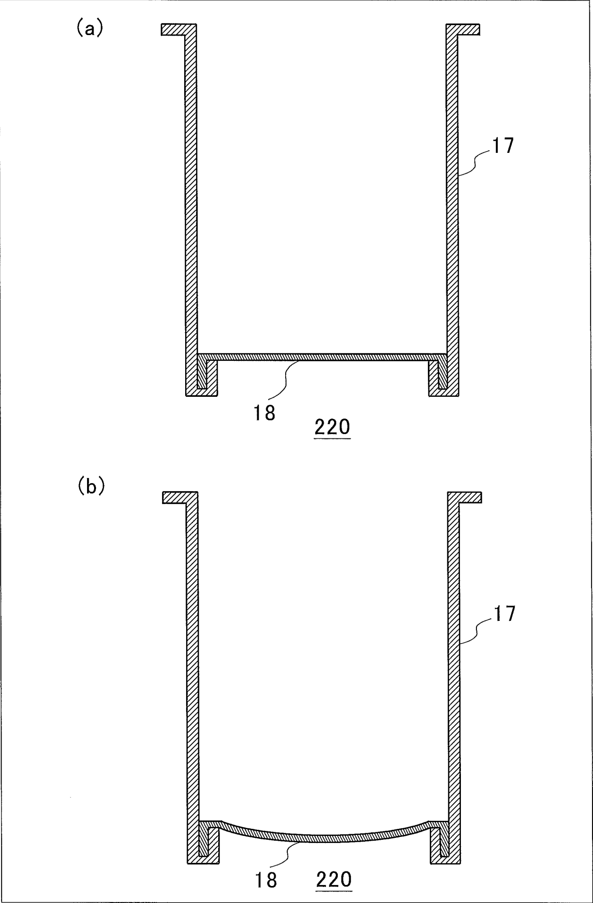
FIG.35
