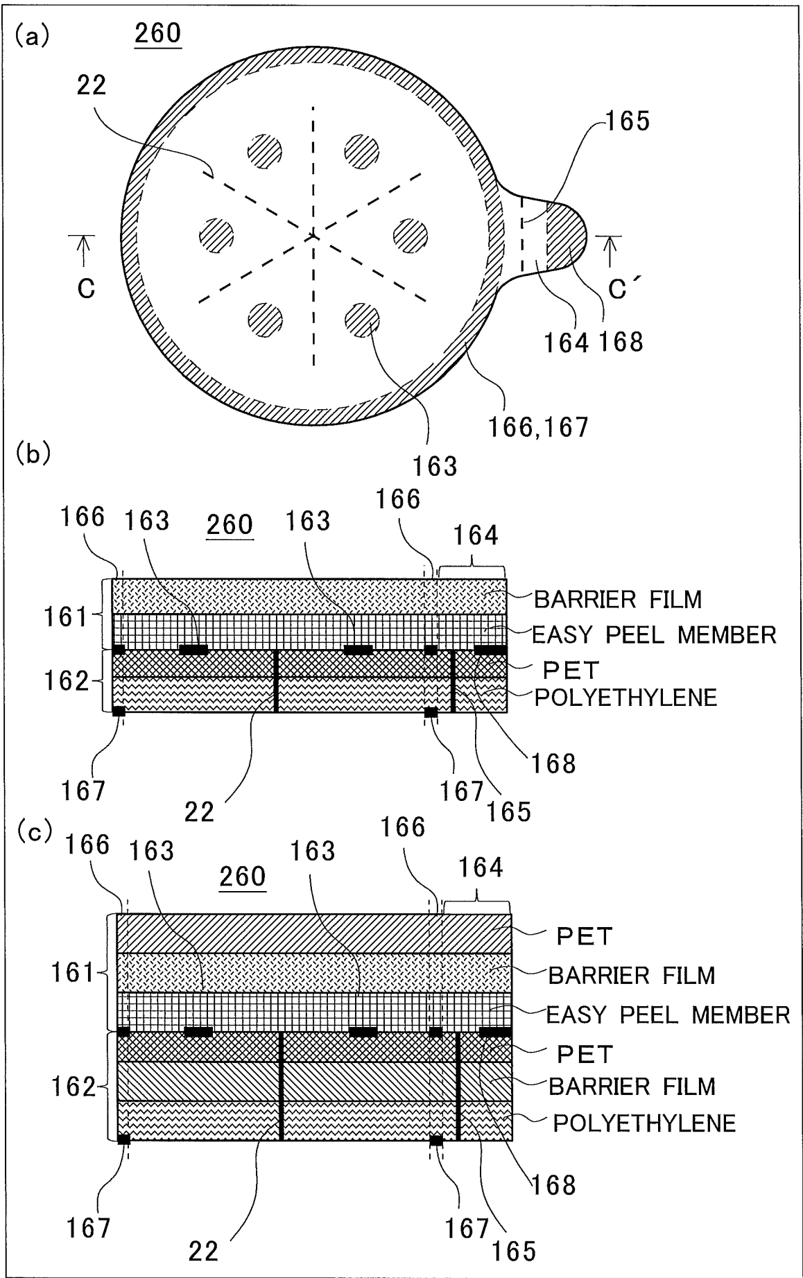
FIG.18
