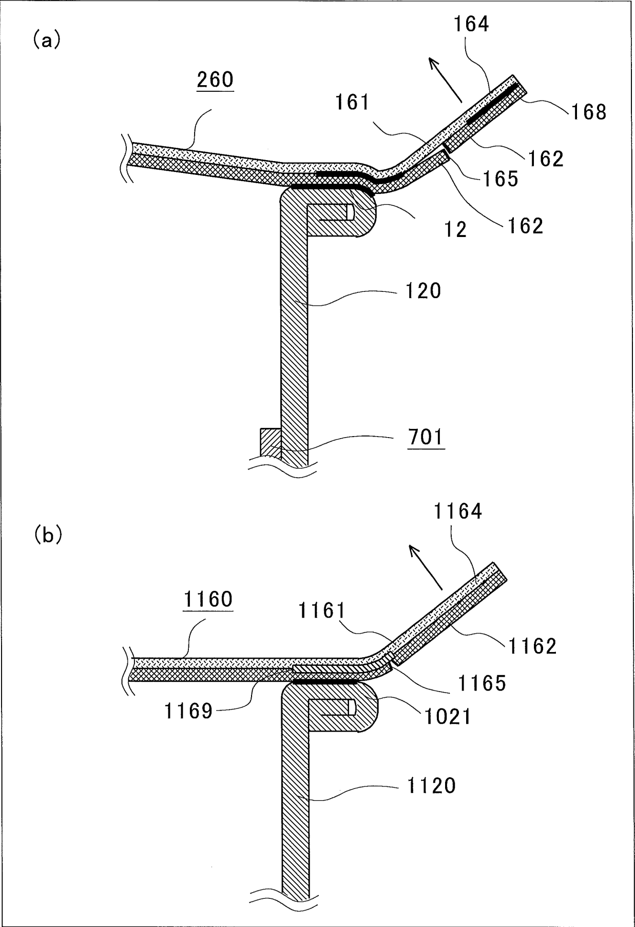
FIG.22
