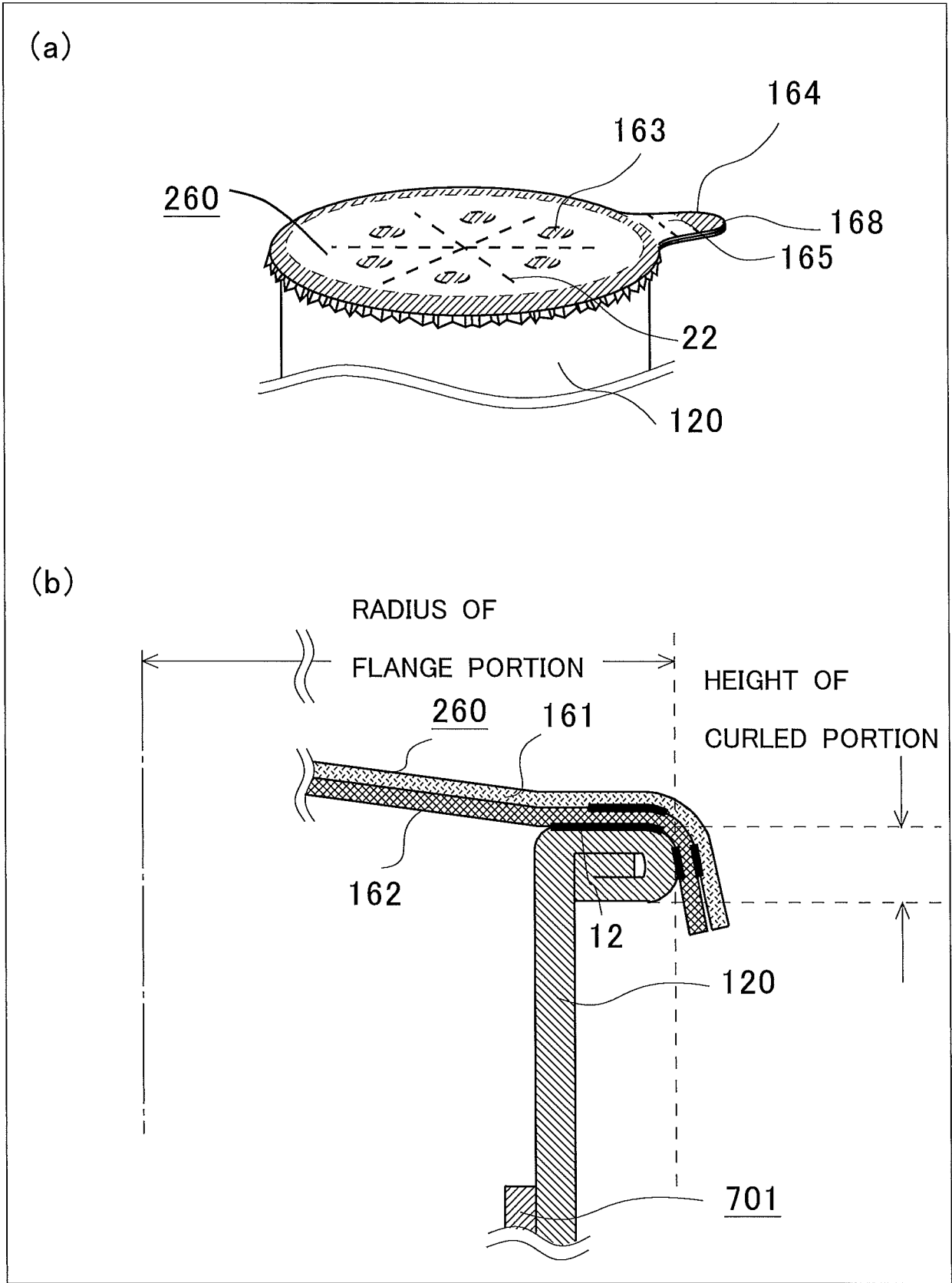
FIG.21
