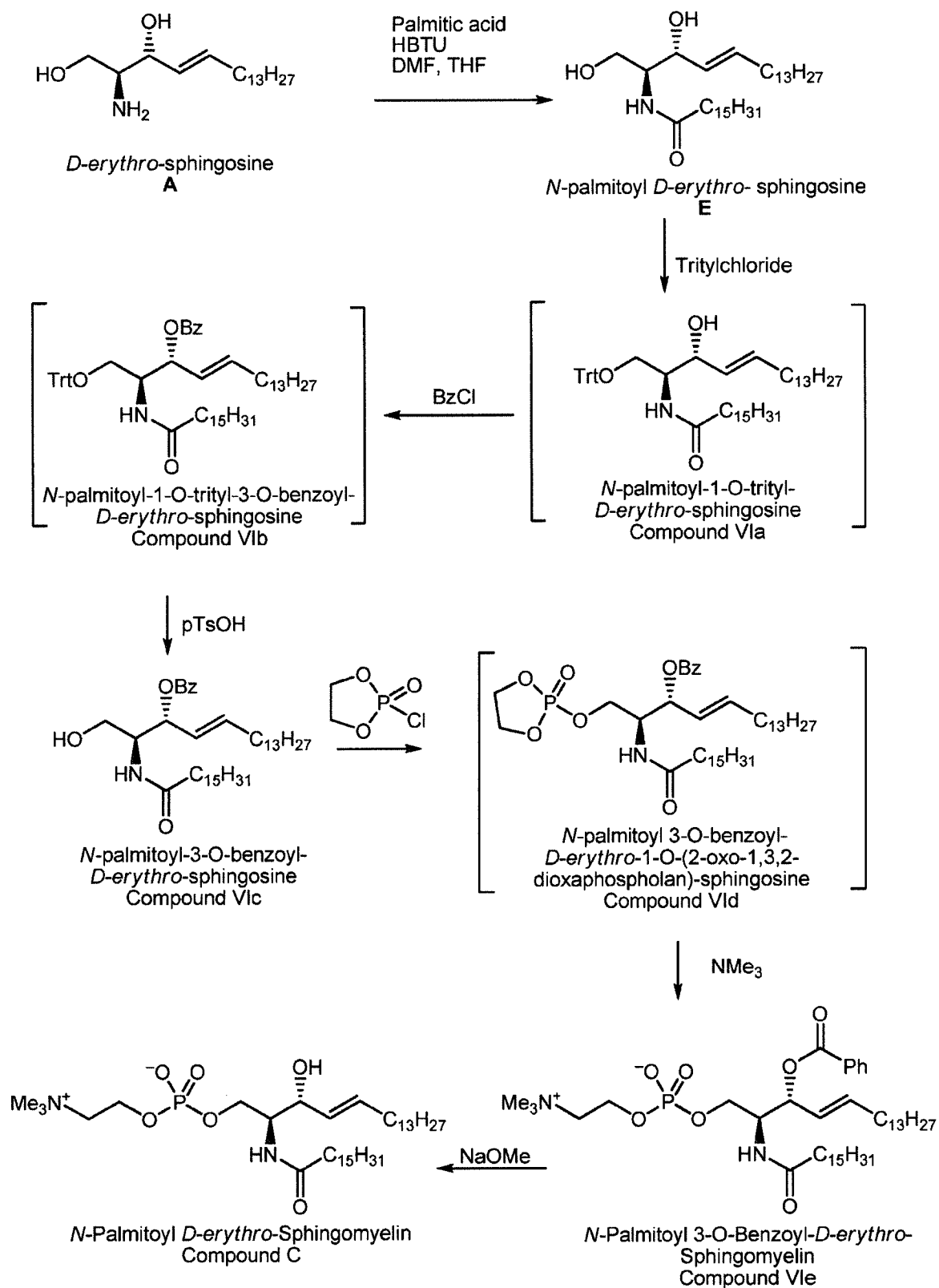
Scheme VI
