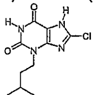
b) 8-chloro-3-(3-methylbutyl)-3,7-dihydro-1H-purine-2,6-dione
