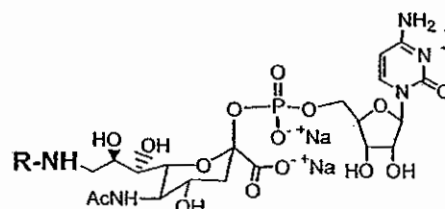
CMP-NeuAc-9-NH-R
