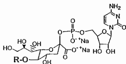
CMP-KDN-5-O-R
