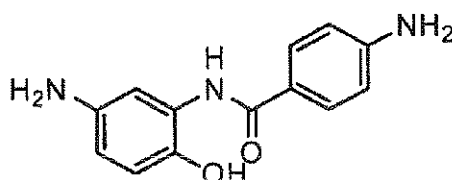
Hydroxyl group-containing diamine (d)
