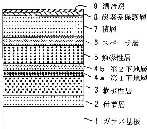
10 垂直磁気記録ディスク
